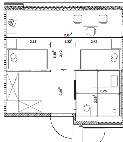
Grundriss-Musterzimmer
