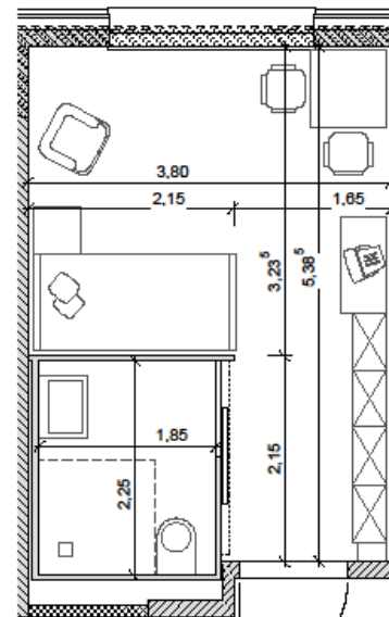
Grundriss-Musterzimmer
